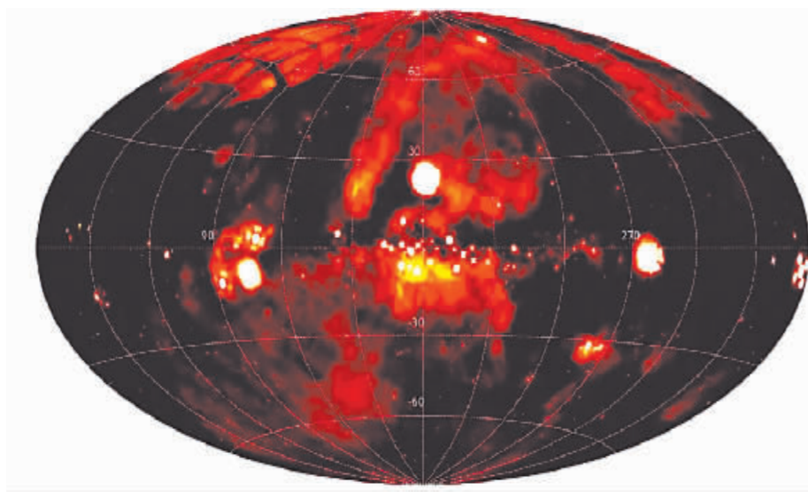
“天关”卫星获取的全天X射线天图。(中国科学院国家天文台供图)
