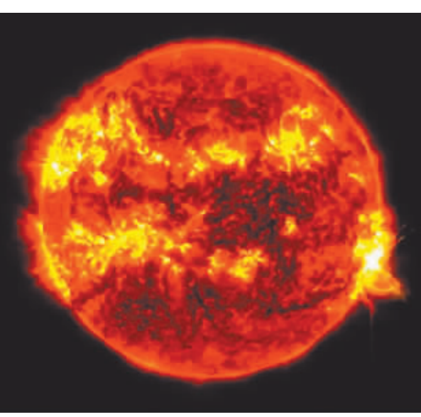
NASA太阳动力学观测站14日拍摄太阳耀斑图像。
