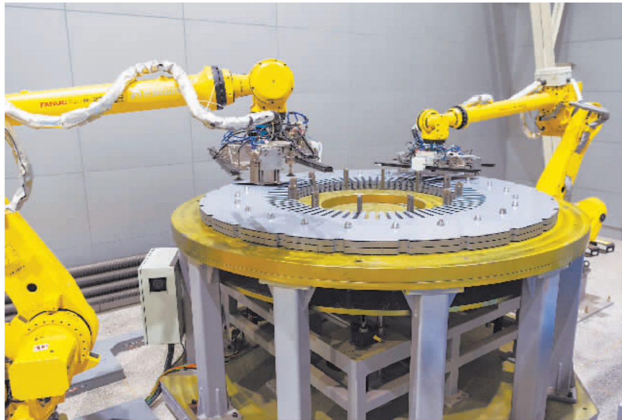
在哈电集团哈尔滨电机厂有限责任公司的生产车间,智能叠片机器人在进行自动化作业。
