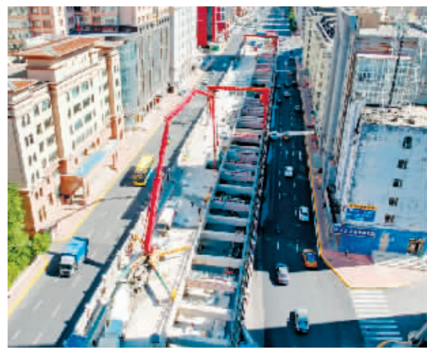
地铁3号线上海街站施工现场。
