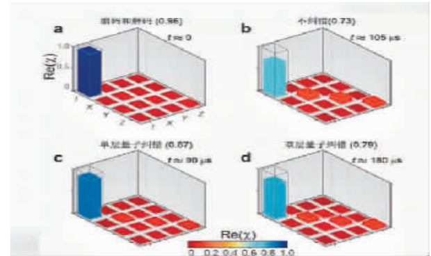
量子纠错操作的实验表征结果。研究团队供图
