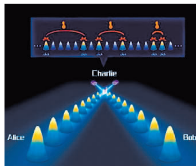
模式匹配量子密钥分发协议示意图。(中国科学技术大学供图)
