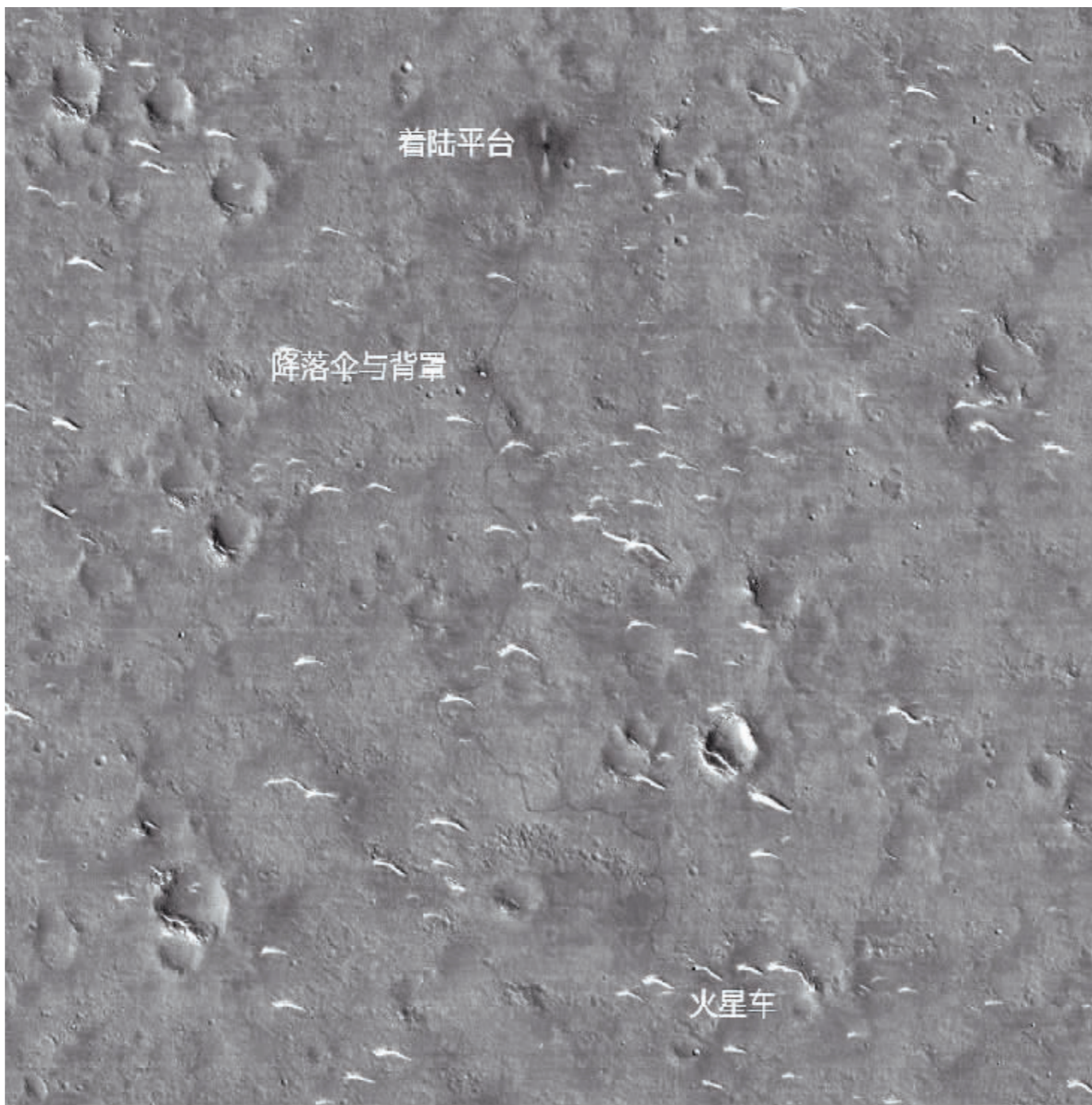
图为高分辨率相机拍摄“祝融号”巡视区影像。
