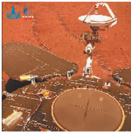
2022年1月22日(着陆后第247火星日),火星车表面存在明显的沙尘覆盖。
