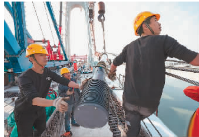
新建福厦铁路安海特大桥建设者正在施工。
